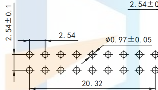
PCB开孔
